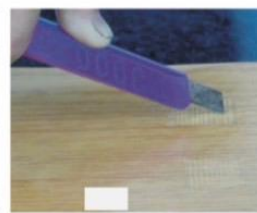
●板面刀割百格試驗 不掀起
